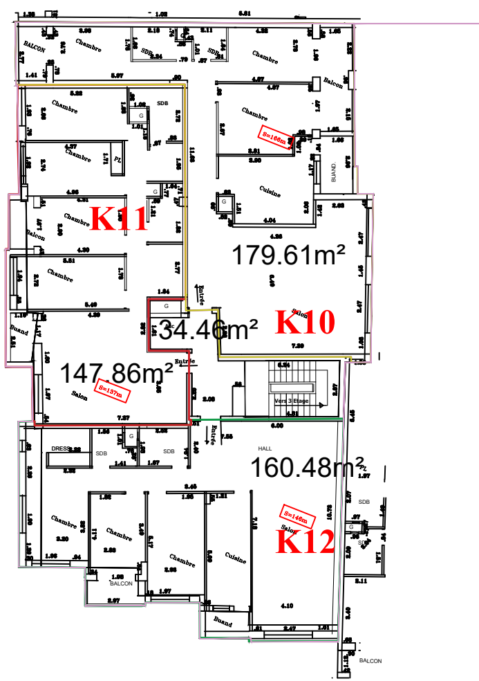
IMM K-1er ETAGE
